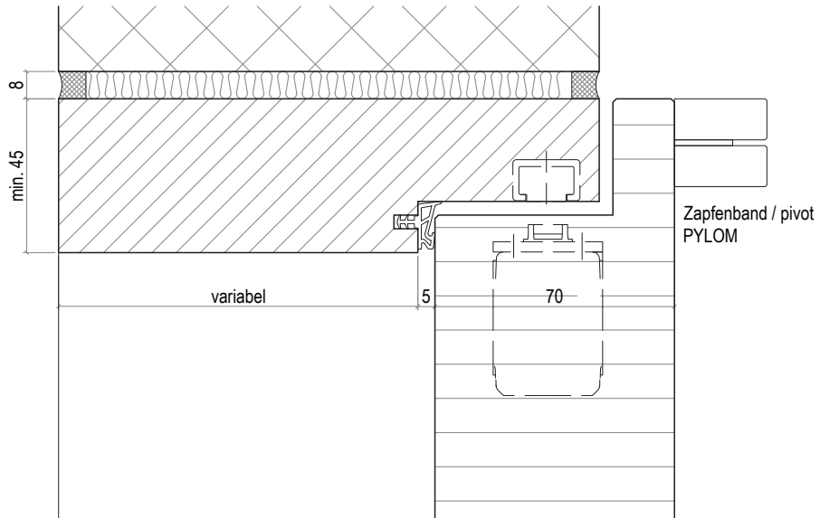
Détail de raccord au plafond (coupe verticale)
