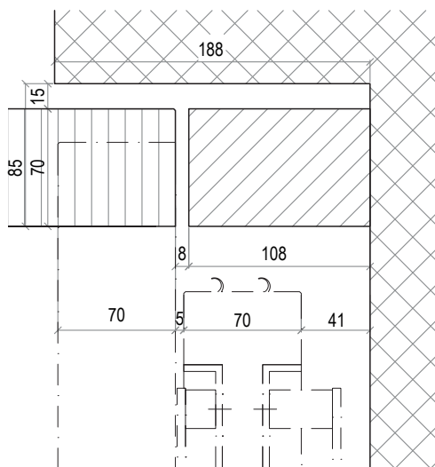
Détail côté pivot et aimant poignée EN179 (coupe horizontale)
