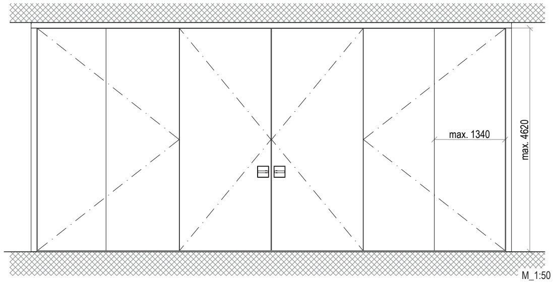
Exécution 2 vantaux 4 parties (élévation)
