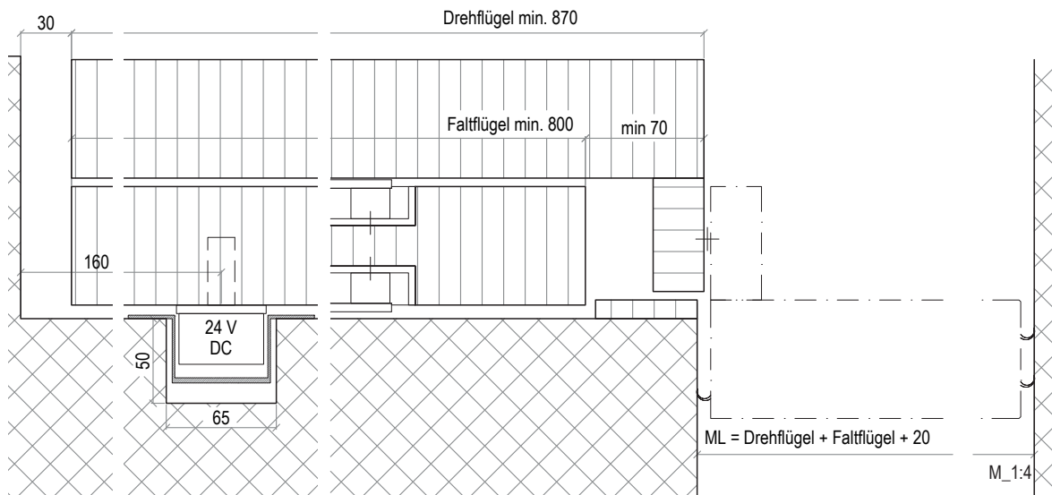
Détails exécution 180° (coupe horizontale)
