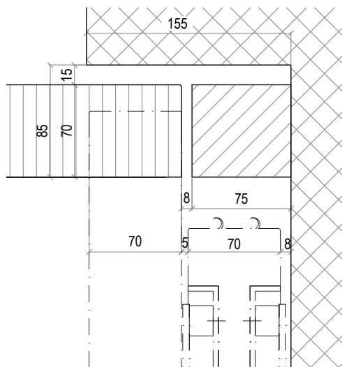
Détail côté pivot et aimant (coupe horizontale)
