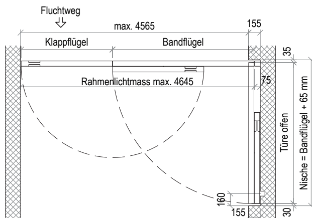
Exécution 1 vantail 90°, 2 parties (coupe horizontale)
