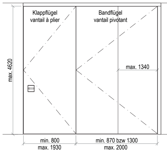
Exécution 1 vantail 2 parties (élévation)
