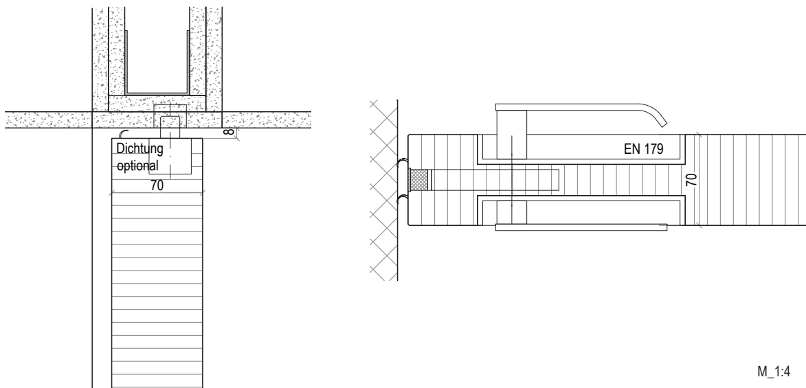
Raccord au plafond variante sans cadre (coupe verticale), variante poignée cuvette (coupe horizontale)
