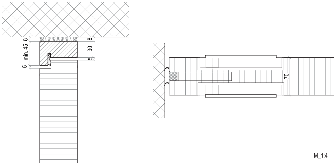
Raccord au plafond et détail serrure (coupe verticale/horizontale)
