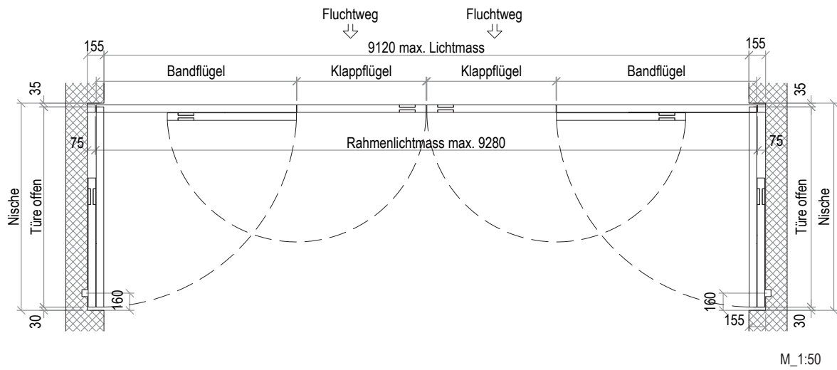
Exécution 2 vantaux 4 parties (coupe horizontale)
