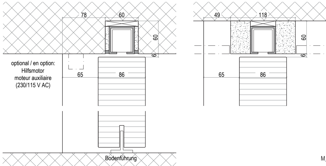
Détail de linteau/détail de sol (coupe verticale)
