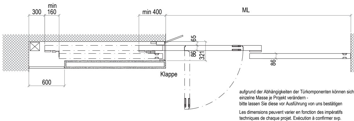
Variante d'exécution télescopique (coupe horizontale)
