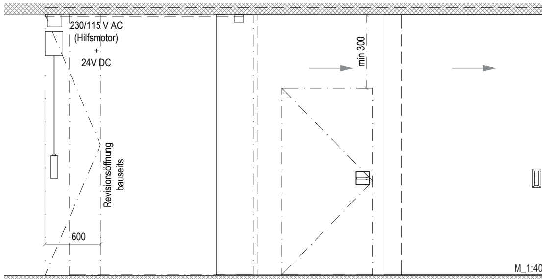
Variante d'exécution télescopique (élévation)
