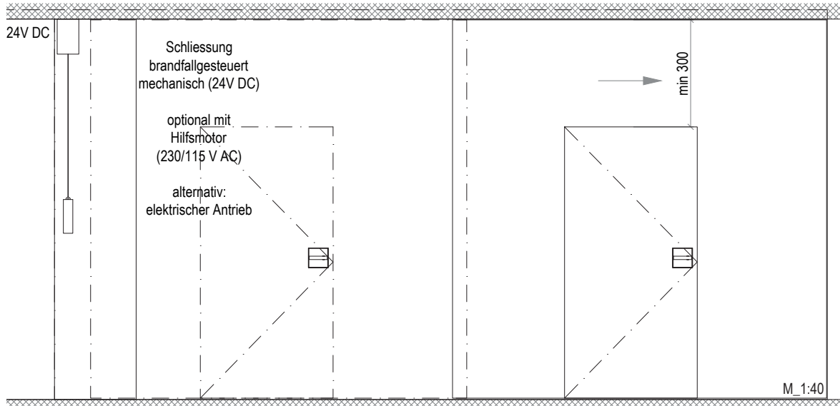
Variante avec porte de fuite (élévation)
