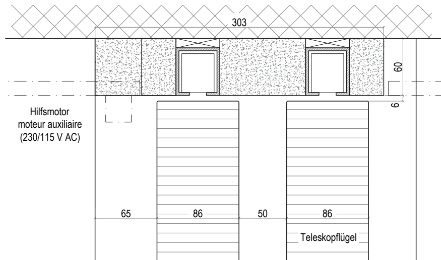
Variante d'exécution (coupe verticale)
