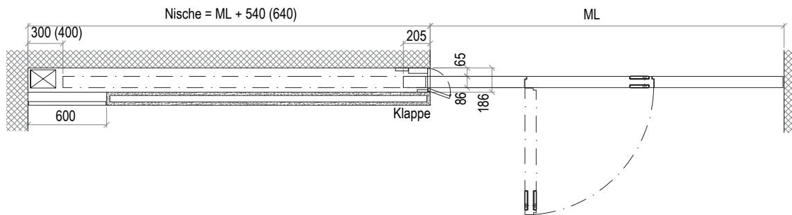
Variante avec porte de fuite, dimensions (coupe horizontale)
